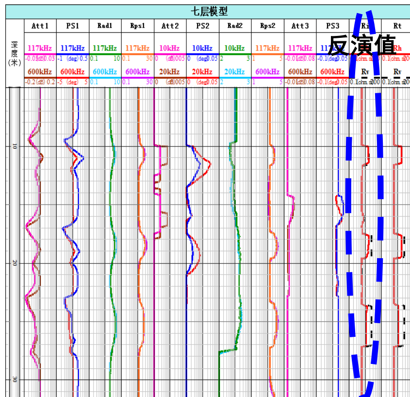
测井响应及基于神经网络的参数提取
