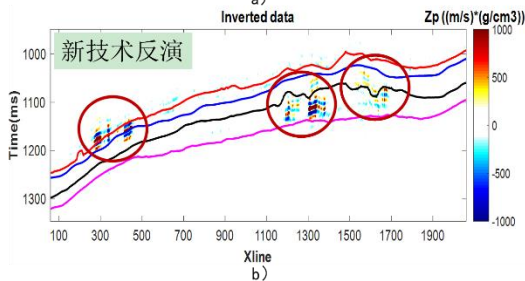
时移地震叠前三参数差异反演技术
