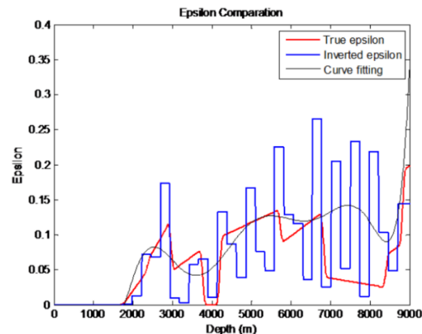
井周 \epsilon 对比
