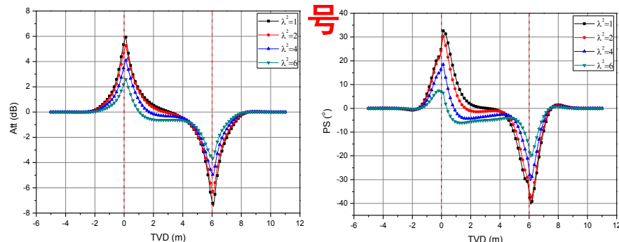
各向异性地层中单发单收仪器方位信号
