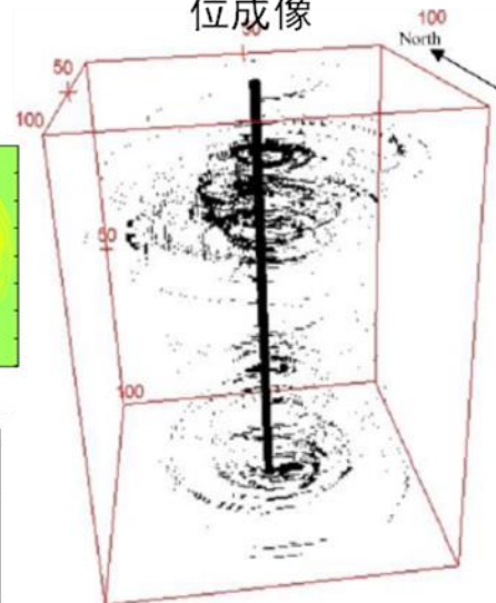
井周反射体三维方位成像
