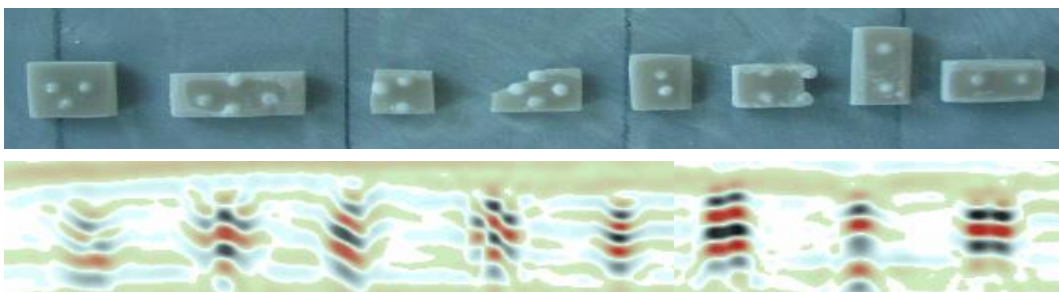
储层特征与地震响应特征的对应关系
