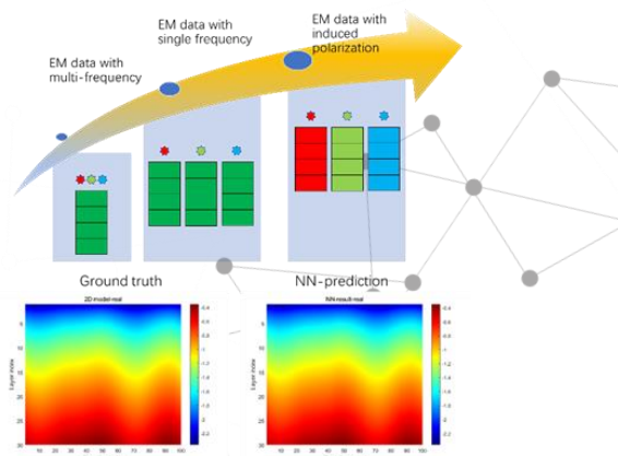
复电阻率反演
