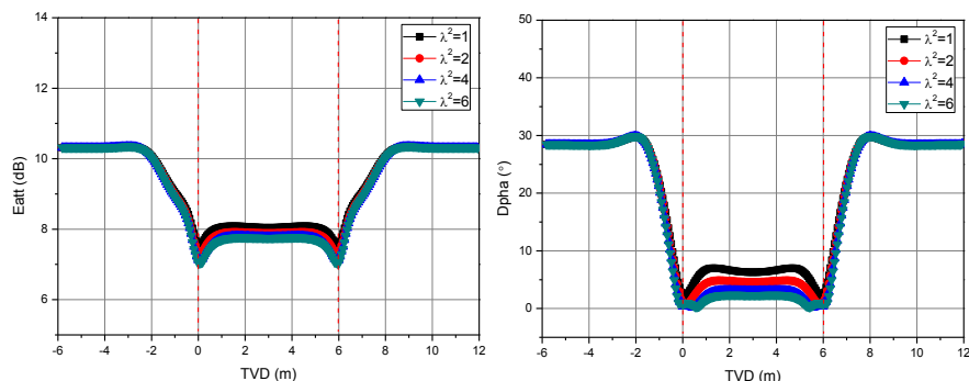
各向异性地层中单发双收仪器常规信号
