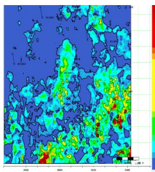
实际资料孔隙渗透率预测
