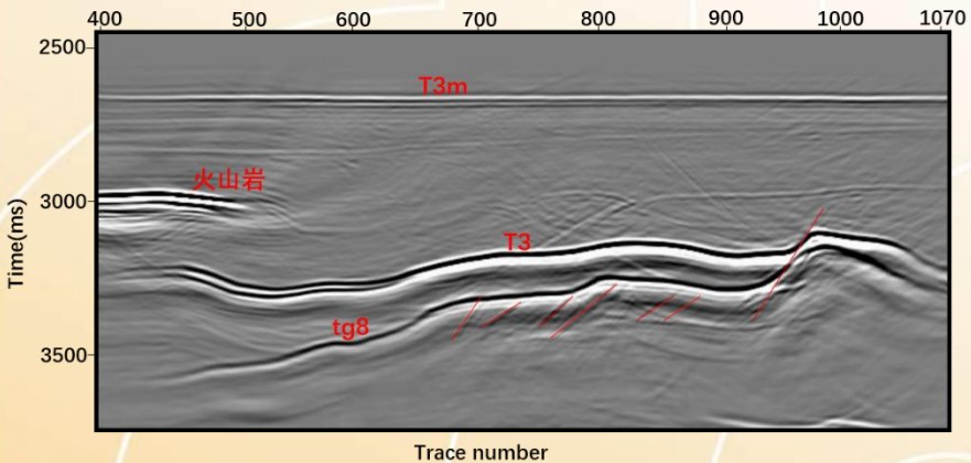
240线成果剖面
