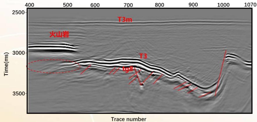
600线成果剖面
