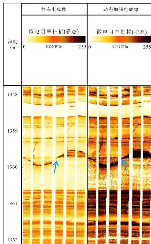
图5 J13井成像测井中的构造裂缝(井位图如图1c所示，箭头指示裂缝)
