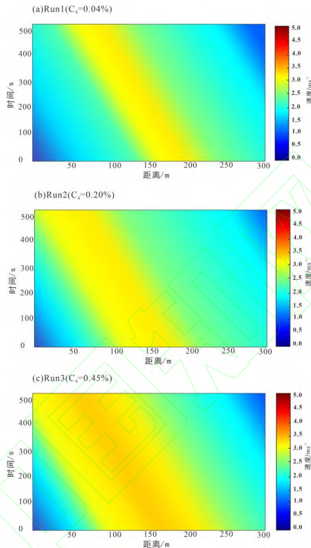
图2 浊流流速剖面图(图a、b、c为Run1、Run2、Run3流速分布)
