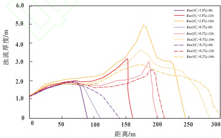
图5 Run1、Run2、Run3 在 80 s、120 s、160 s 时沿程浊流厚度分布图
