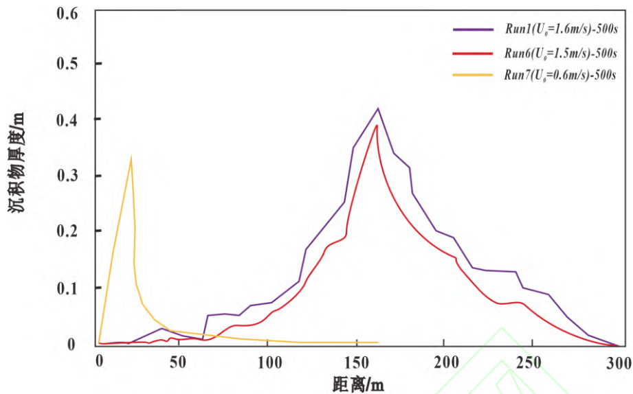
图 14 Run1、Run 6、Run7 模拟结束沿程沉积物厚度分布图
