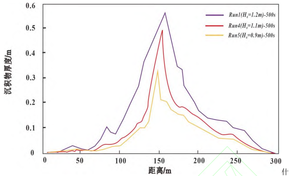
图 11 Run1、Run 4、Run5 模拟结束沿程沉积物厚度分布图
