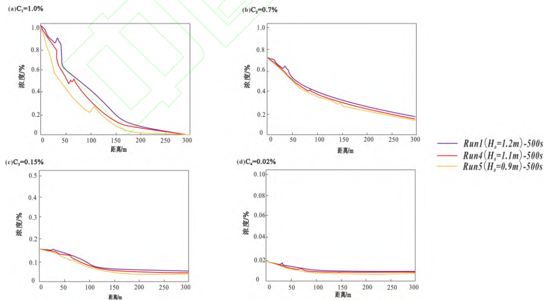
图 10 Run1、Run 4、Run5 模拟结束沿程各颗粒浓度分布图
