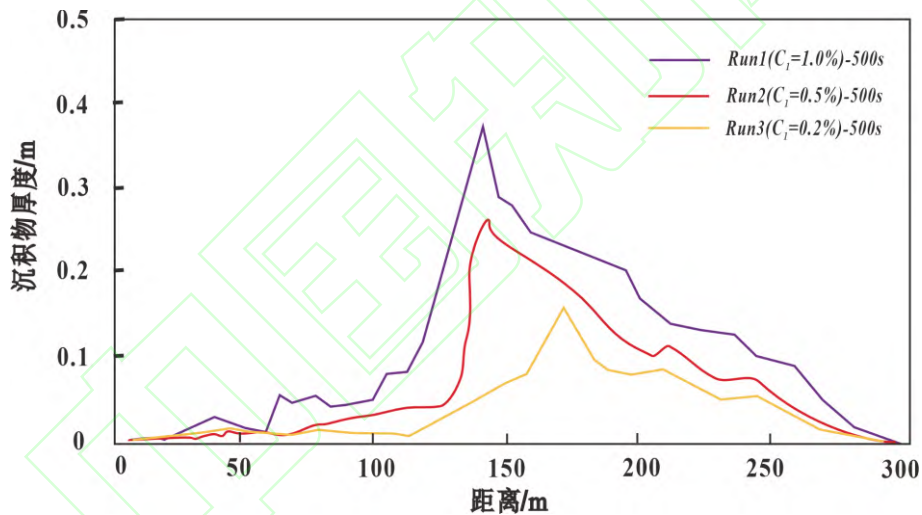
图7 Run1、Run2、Run3 在 500s 时沿程沉积物分布图
