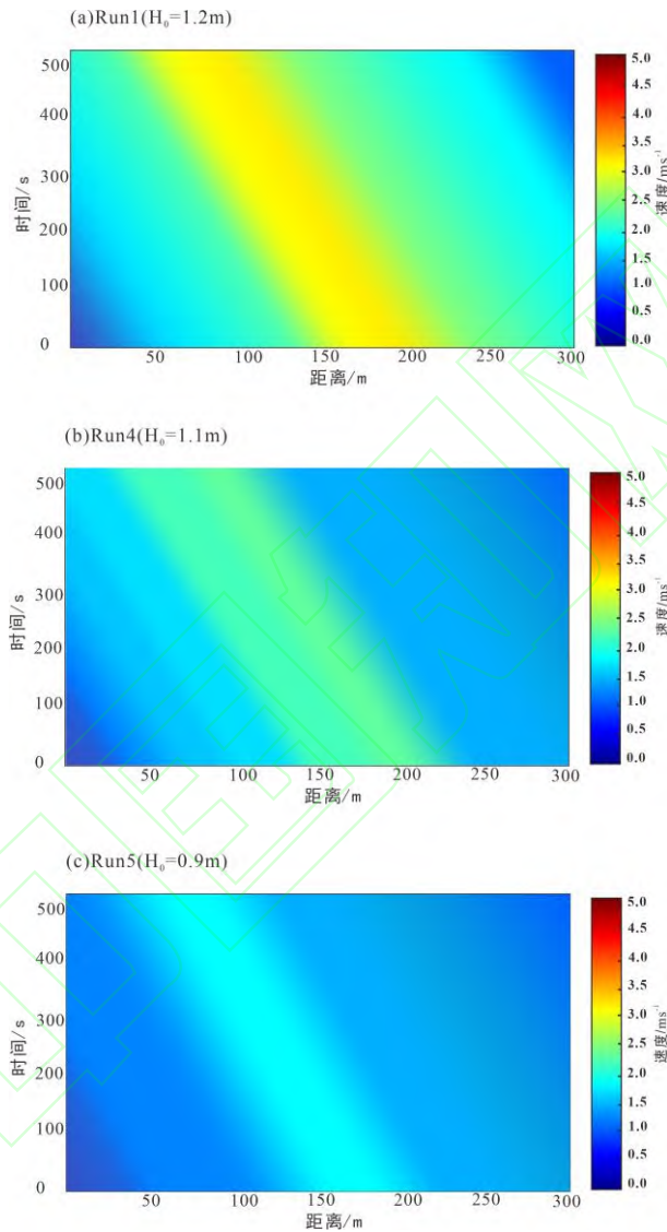
图 8 浊流流速剖面图（图 a、b、c 为 Run1、Run4、Run5 流速分布）
