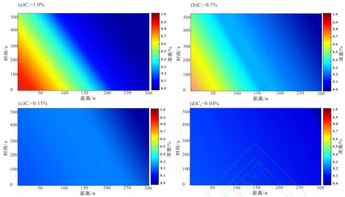
图6 Run1 中各颗粒浓度沿程剖面图
