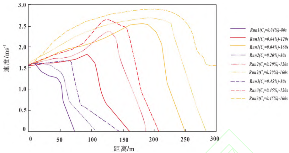
图3 Run1、Run2、Run3 在 80s、120s、160s 时沿程速度分布图
