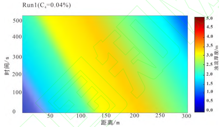
图4 浊流厚度沿程剖面图
