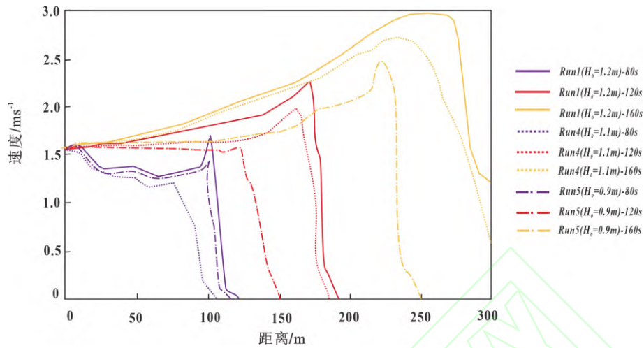
图9 Run1、Run 4、Run 5 在 80s、120s、160s 时沿程速度分布图
