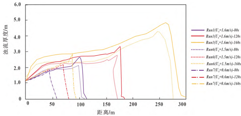
图 12 Run1、Run 6、Run 7 在 80s、120s、160s 时沿程浊流厚度分布图
