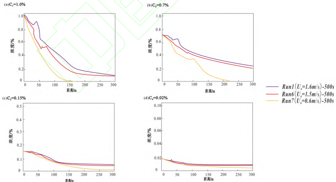
图 13 Run1、Run 6、Run7 模拟结束沿程各颗粒浓度分布图
