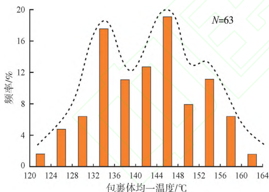
图9 渤中凹陷南部东二下段流体包裹体均一温度分布
