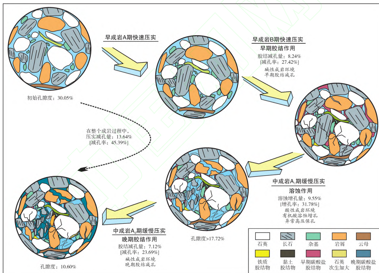
图 11 渤中凹陷南部东二下段湖底扇砂岩储层孔隙综合演化模式
