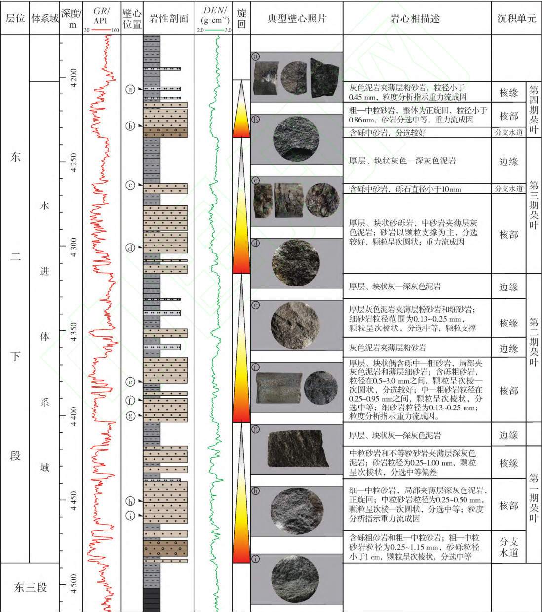
图2 渤中凹陷南部东二下段湖底扇沉积特征(A3井)
