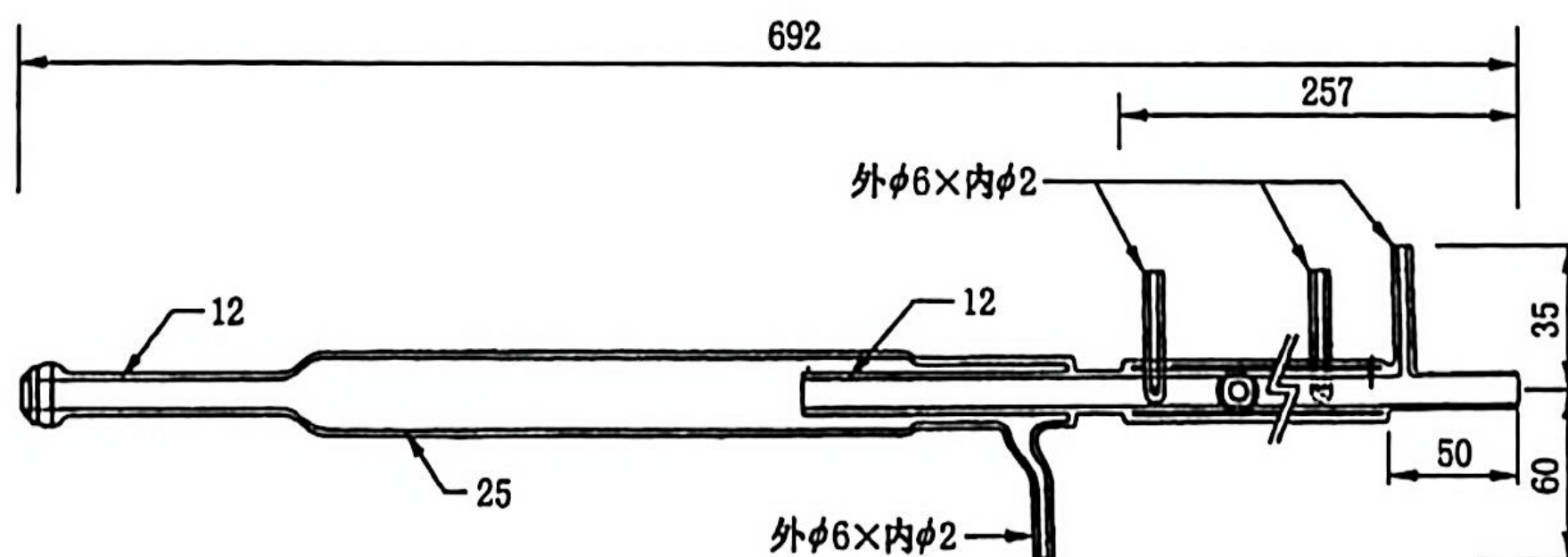
图 2 舟进样燃烧管
