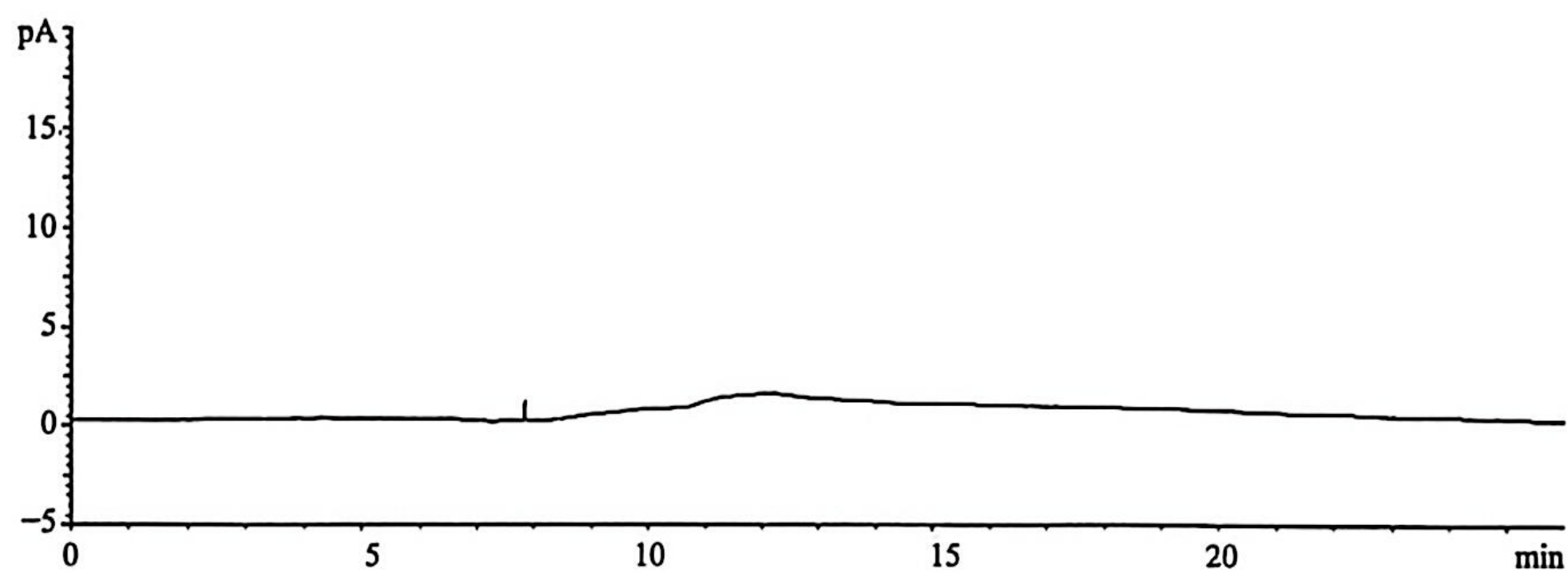
图 B.2 本标准条件下扣除柱补偿后的参考色谱图
