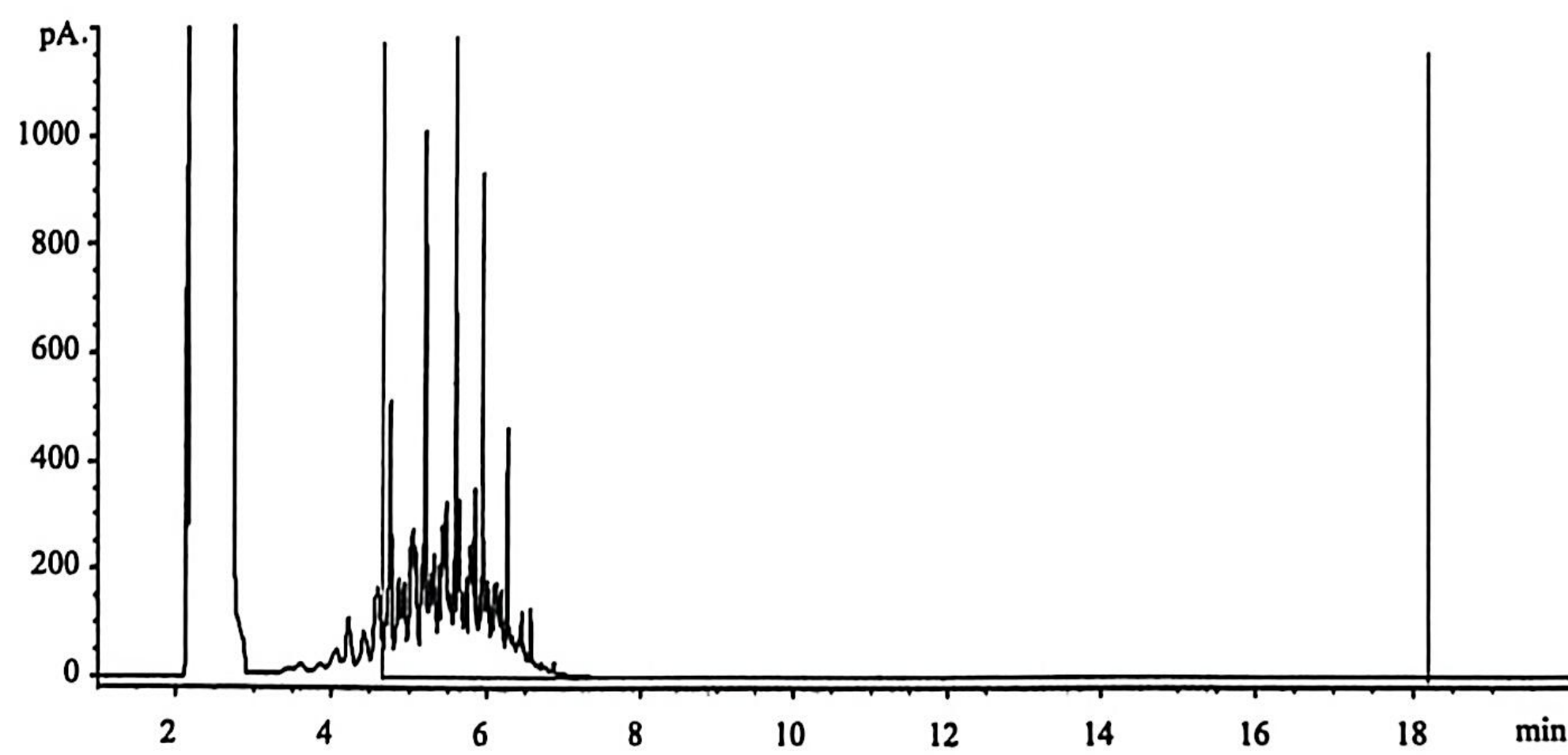
图 B.6 煤油参考色谱图
