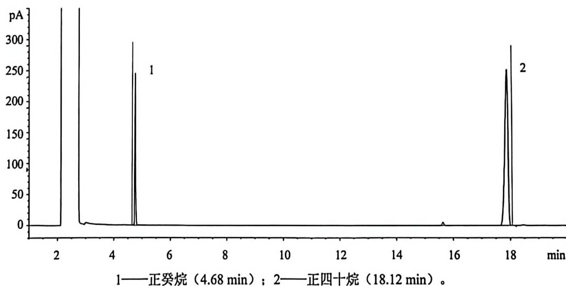
图 1 正癸烷和正四十烷的参考色谱图
