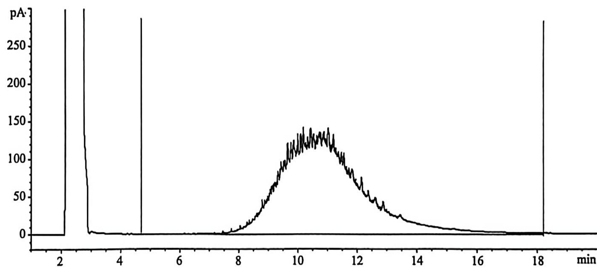
图 B.8 润滑油参考色谱图
