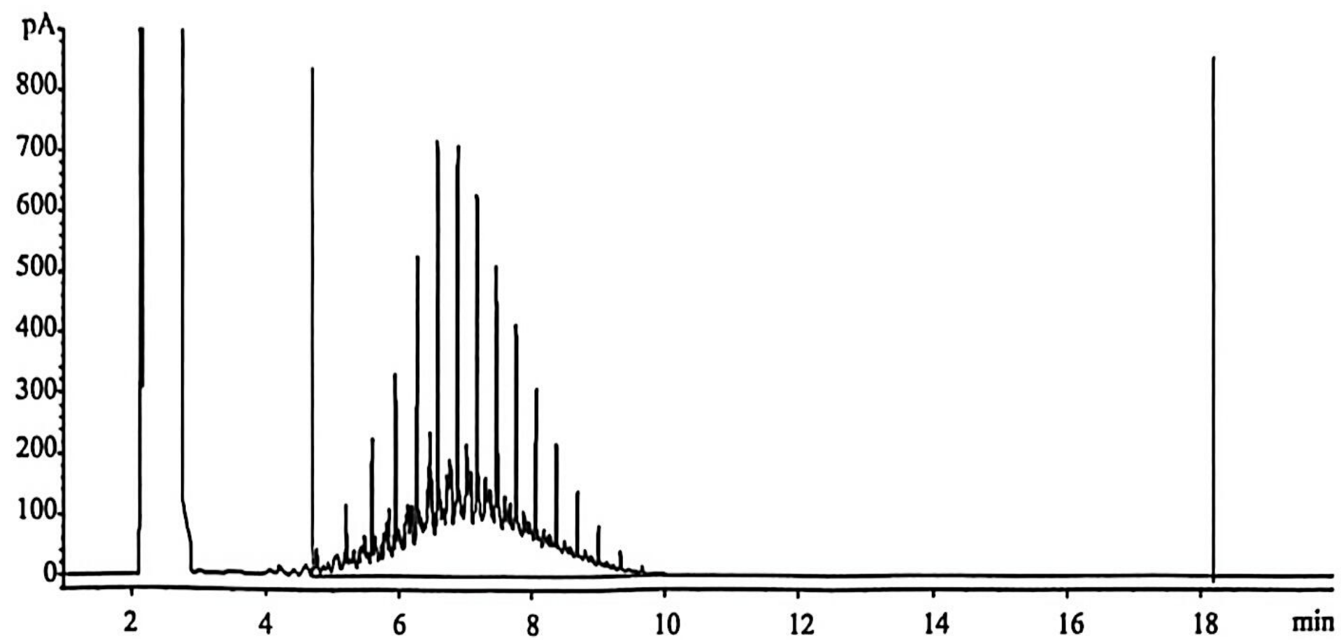
图 B.7 轻柴油参考色谱图
