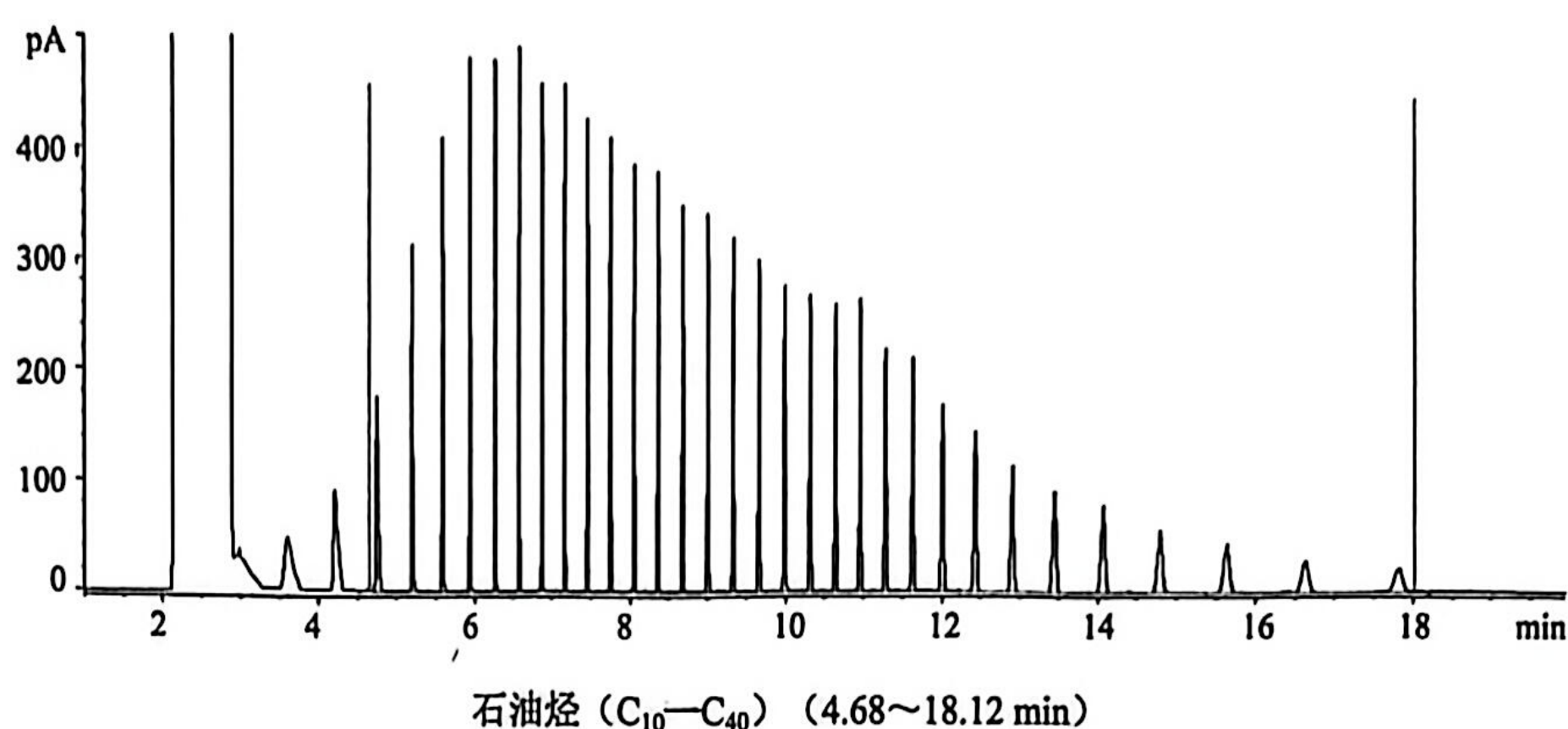
图2 石油烃 (C 10 —C 40 ) 参考色谱图
