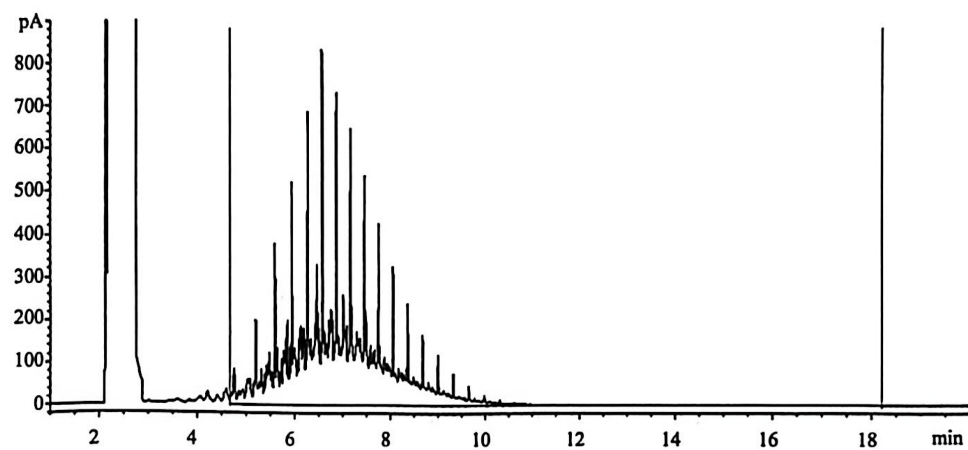
图 B.5 10#柴油参考色谱图
