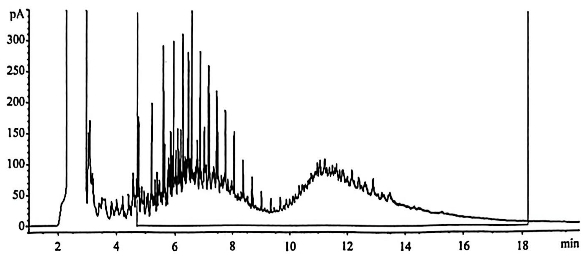
图 B.4 柴油-润滑油（1+1）混合参考色谱图
