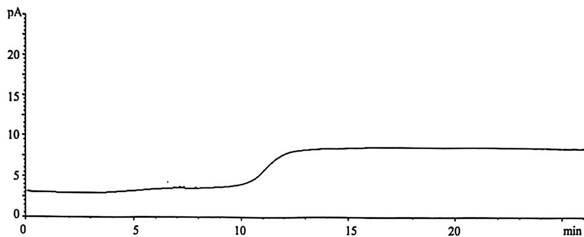
图 B.1 本标准程序升温条件下的柱补偿参考色谱图
