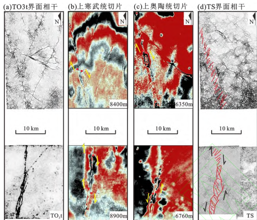
图 8 F 15 断裂水平切片 Fig.8 F 15 fault horizontal section
