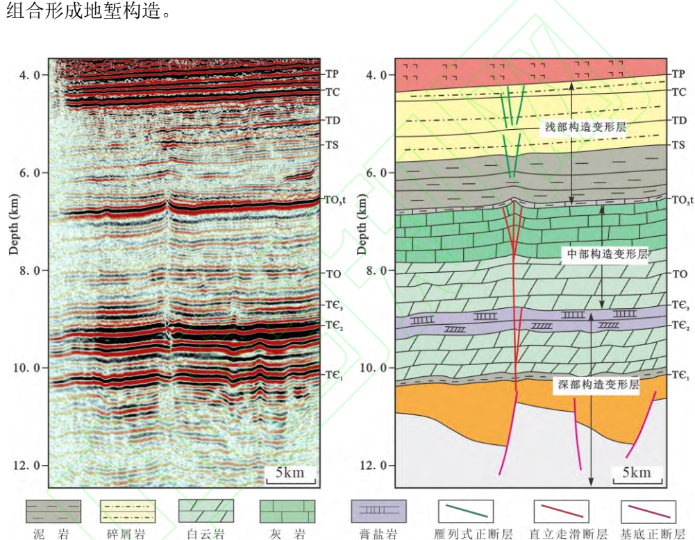
图 5 塔里木盆地富满油田走滑断裂分层差异变形结构
