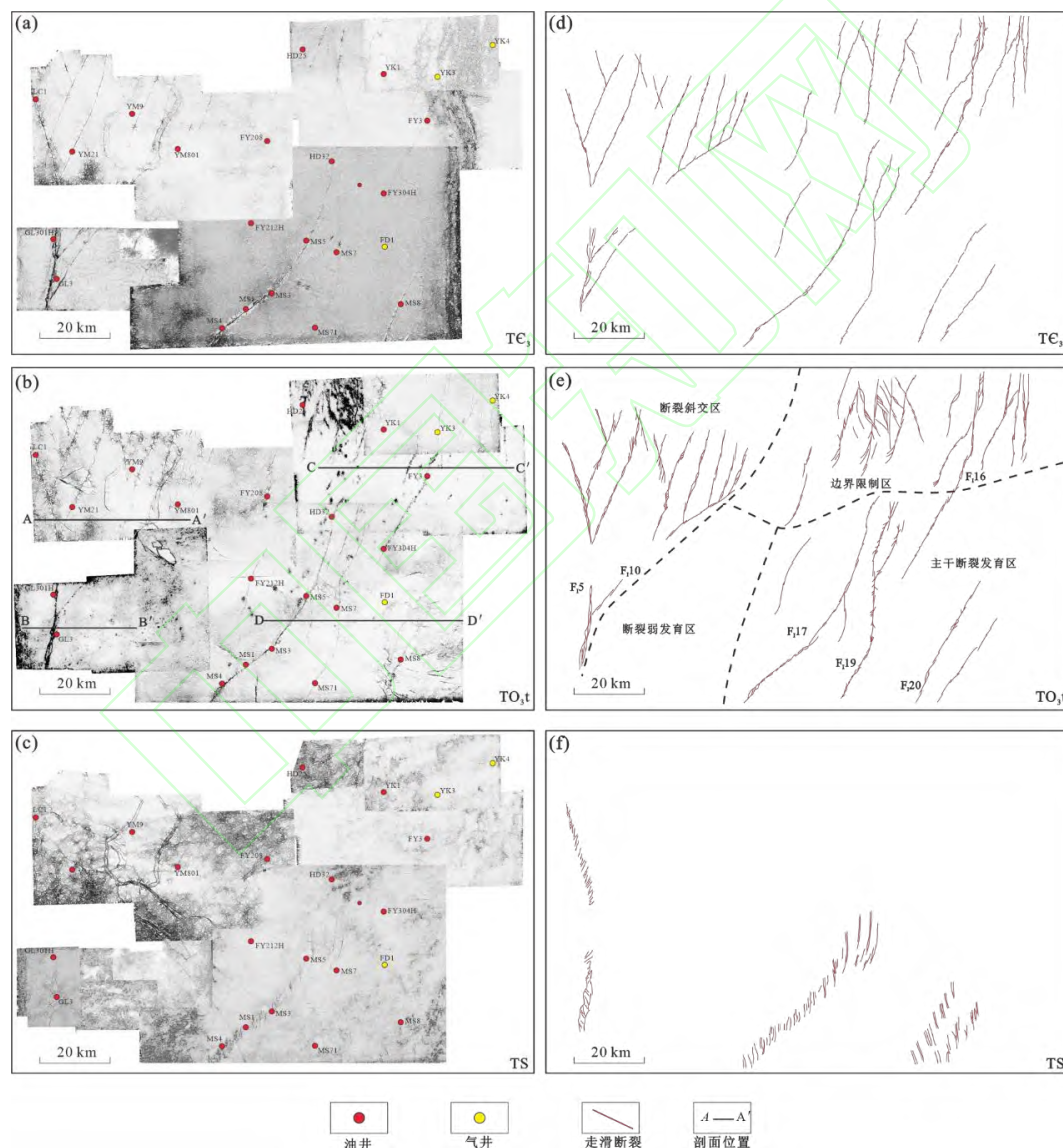
图 4 塔里木盆地富满油田走滑断裂平面特征图(a)上寒武统底面相干；(b)奥陶系一间房组顶面相干；(c)志留系底面相干；(d)上寒武统底面断裂展布特征；(e)奥陶系一间房组顶面断裂展布特征；(f)志留系底面断裂展布特征
