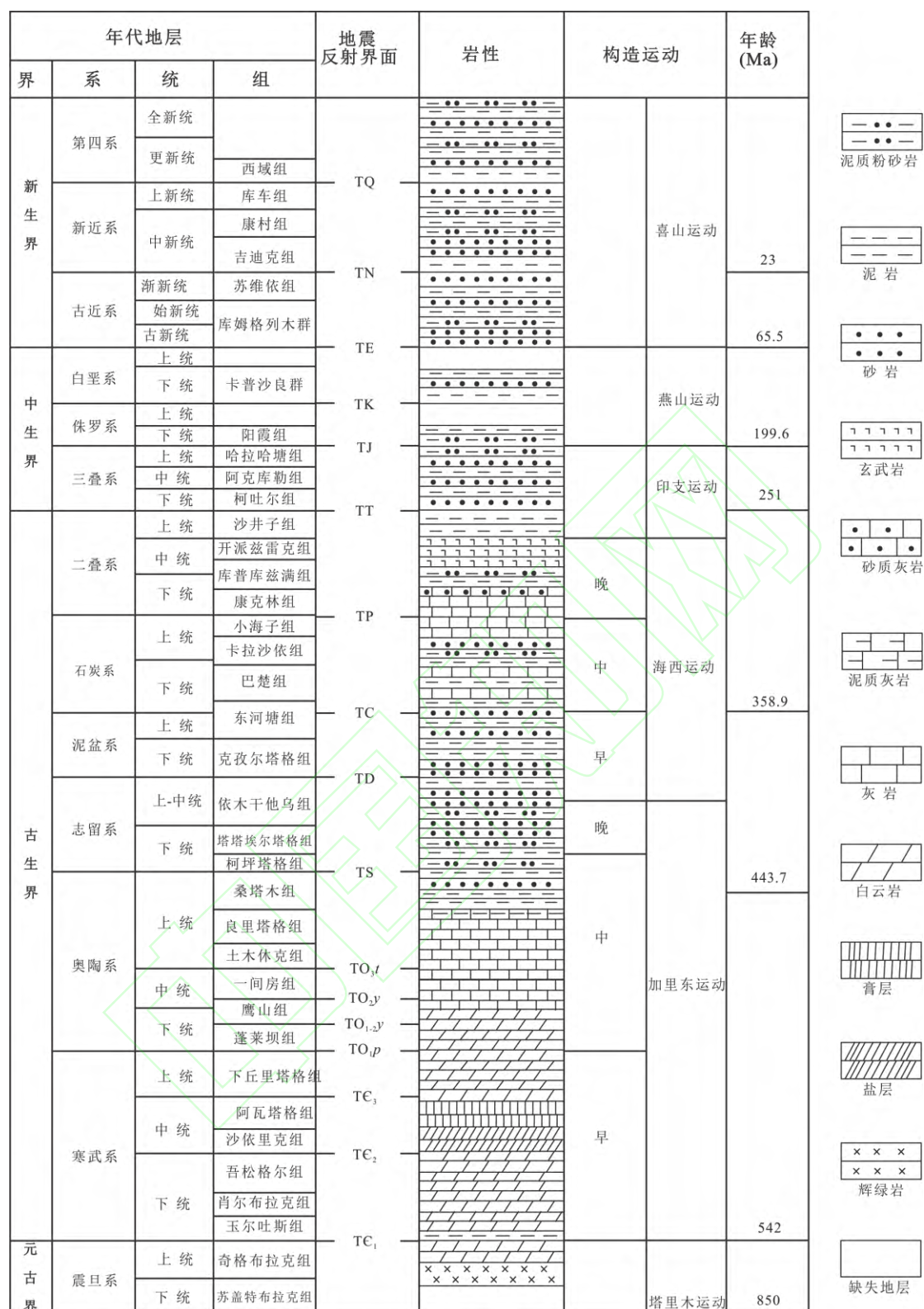
图3 富满油田及邻区地层格架
