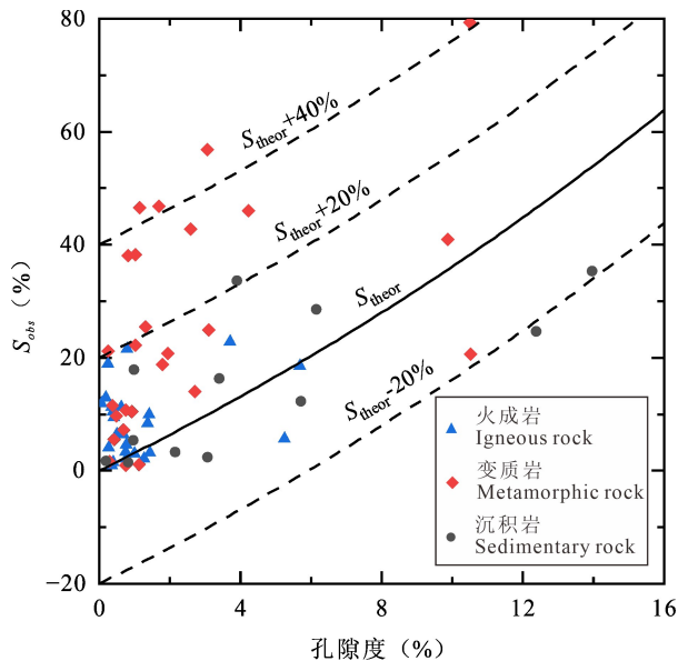
图 7 海南岛孔隙度与影响因子关系图
