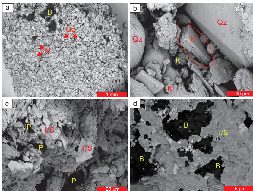
图6 麦克河区块上麦克默里组代表性油砂的扫描电镜图(a为油砂的全貌,部分存在黑色沥青;b为杂基中分布的高岭石矿物;c为杂基中分布的伊蒙混层;d为杂基中粘土矿物吸附了大量沥青;图中B:沥青;Qz:石英;M:杂基;KI:高岭石;P:孔隙;I/S:伊蒙混层)
