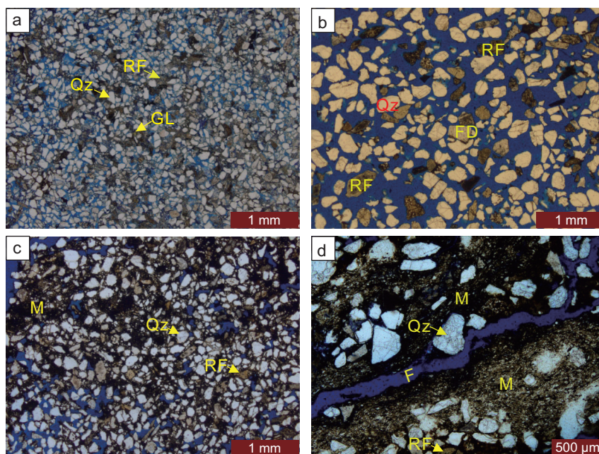
图 4 麦凯河区块上麦克默里组的典型油砂显微图(a. 极细砂岩; b. 细砂岩; c. 杂砂岩; d. 粉砂岩; 图中 B: 沥青; Qz: 石英; M: 杂基; RF: 岩屑; FD: 长石; F: 微裂缝)
