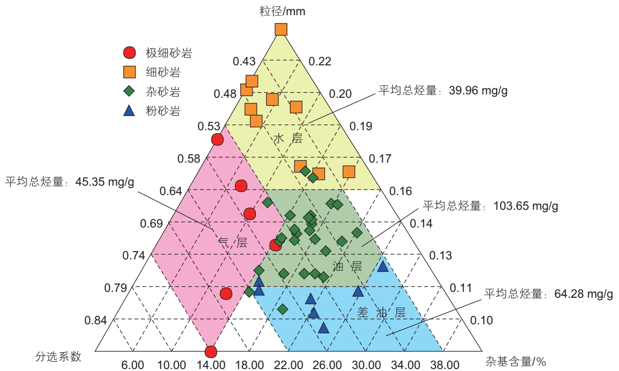
图 11 依据粒径、分选和杂基含量划分麦凯河区块上麦克默里组油砂的含油性图版
