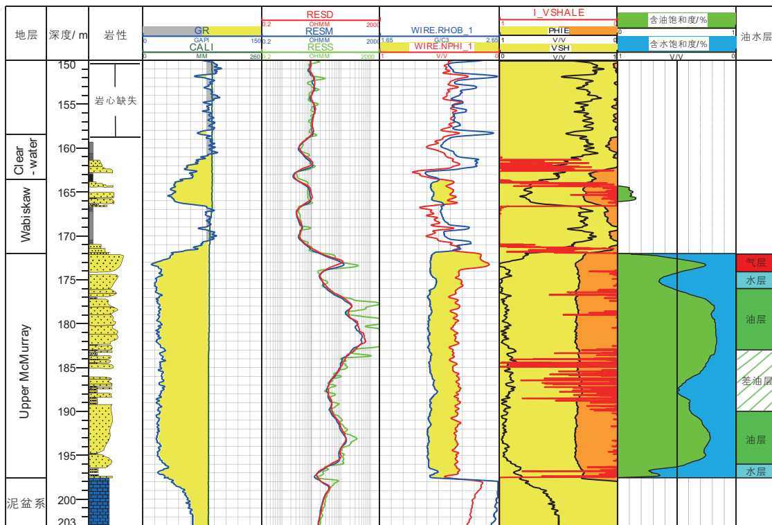
图 9 麦凯河区块上麦克默里组油砂储层评价及油水层划分
