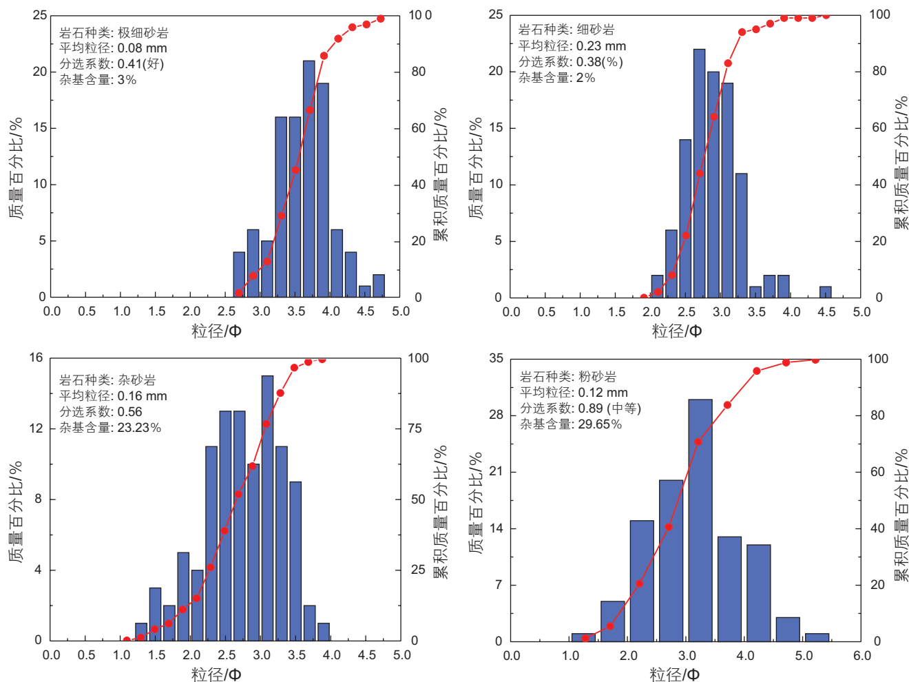
图5 麦凯河区块上麦克默里组4种不同结构油砂的粒度累计曲线和直方图
