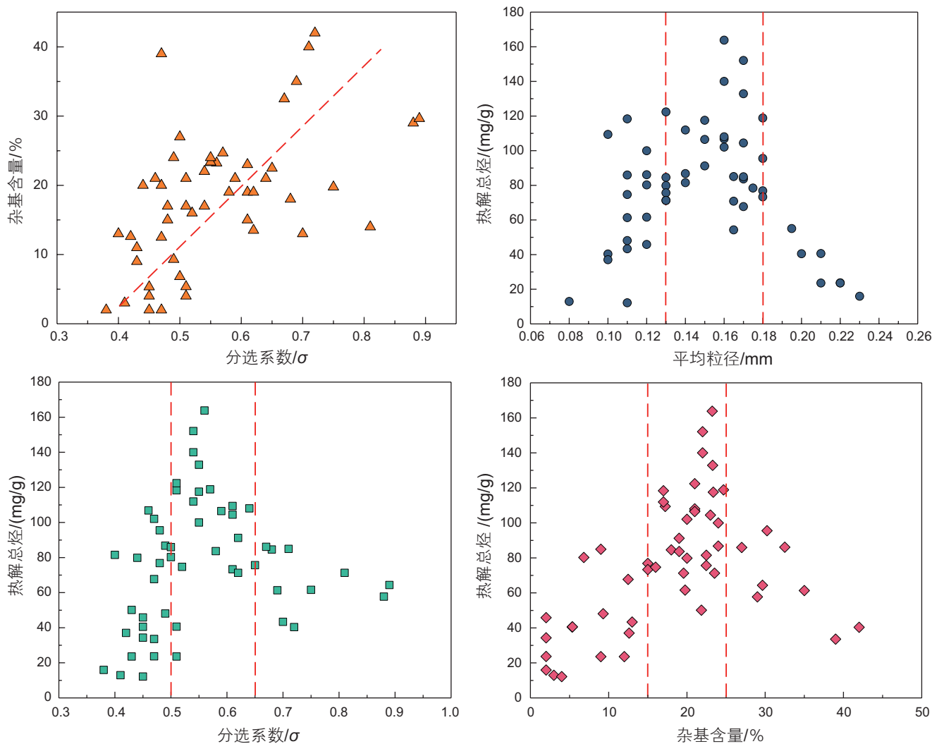
图 10 麦凯河区块上麦克默里组油砂含油性、粒径、分选和杂基含量的相关性
