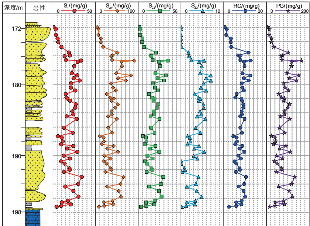
图 8 麦凯河区块上麦克默里组油砂热解组分含量垂向分布特征
