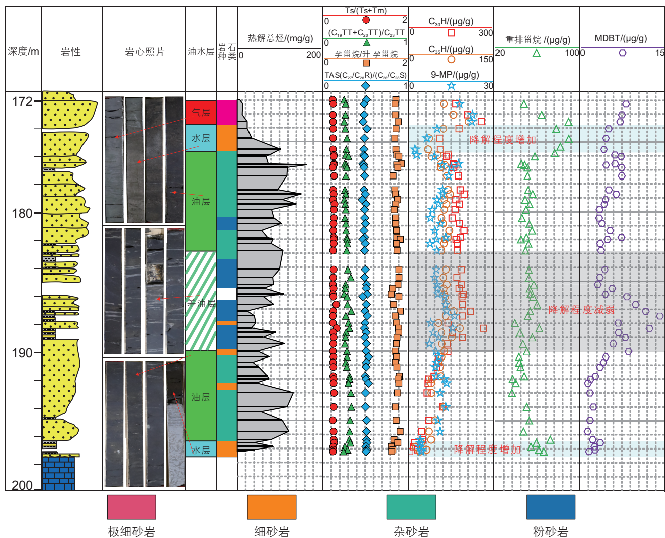
图 14 麦凯河区块上麦默里组岩石类型与含烃量、降解程度和油水层分布的关系
