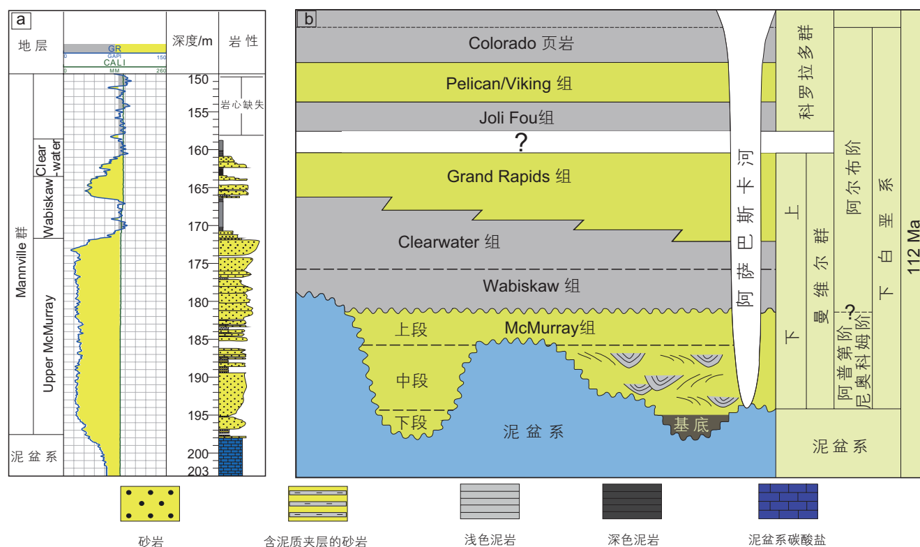
图 2 阿萨巴斯卡地区的 stratigraphic 分布图 (b) 和麦凯河区块麦默里组油砂的层位 (a)
