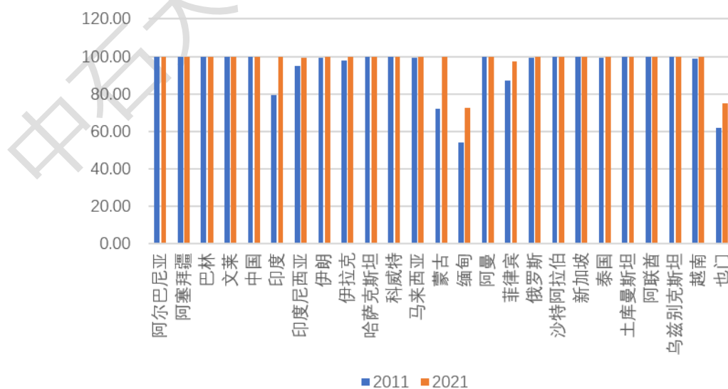
图 2 “一带一路”资源国获得电力人口占比分析图
