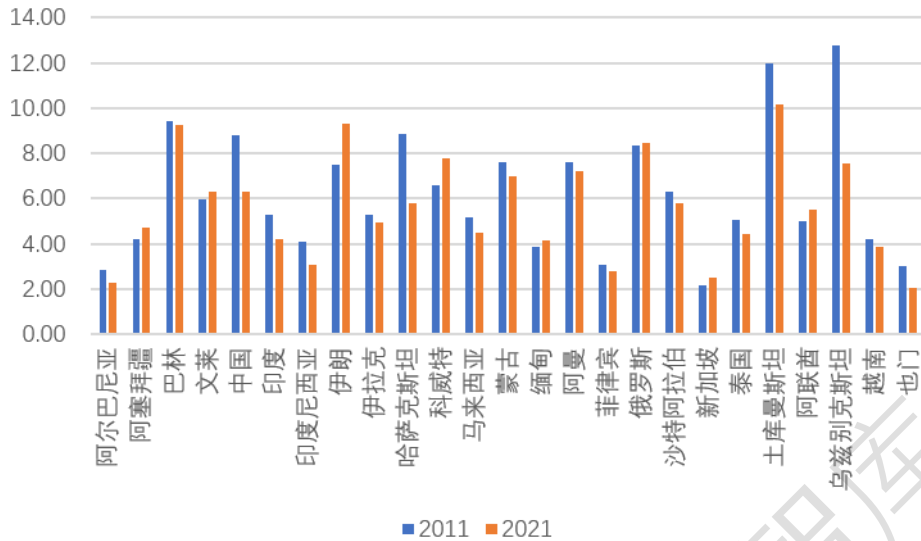
图 3 “一带一路”资源国一次能源强度水平分析图
