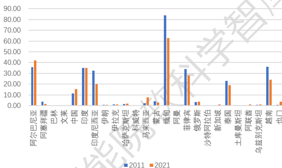
图1 “一带一路”资源国可再生能源消耗量情况分析图
