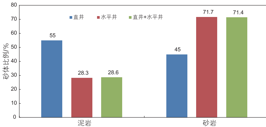
图4 直井与水平井钻遇砂体比例对比图
