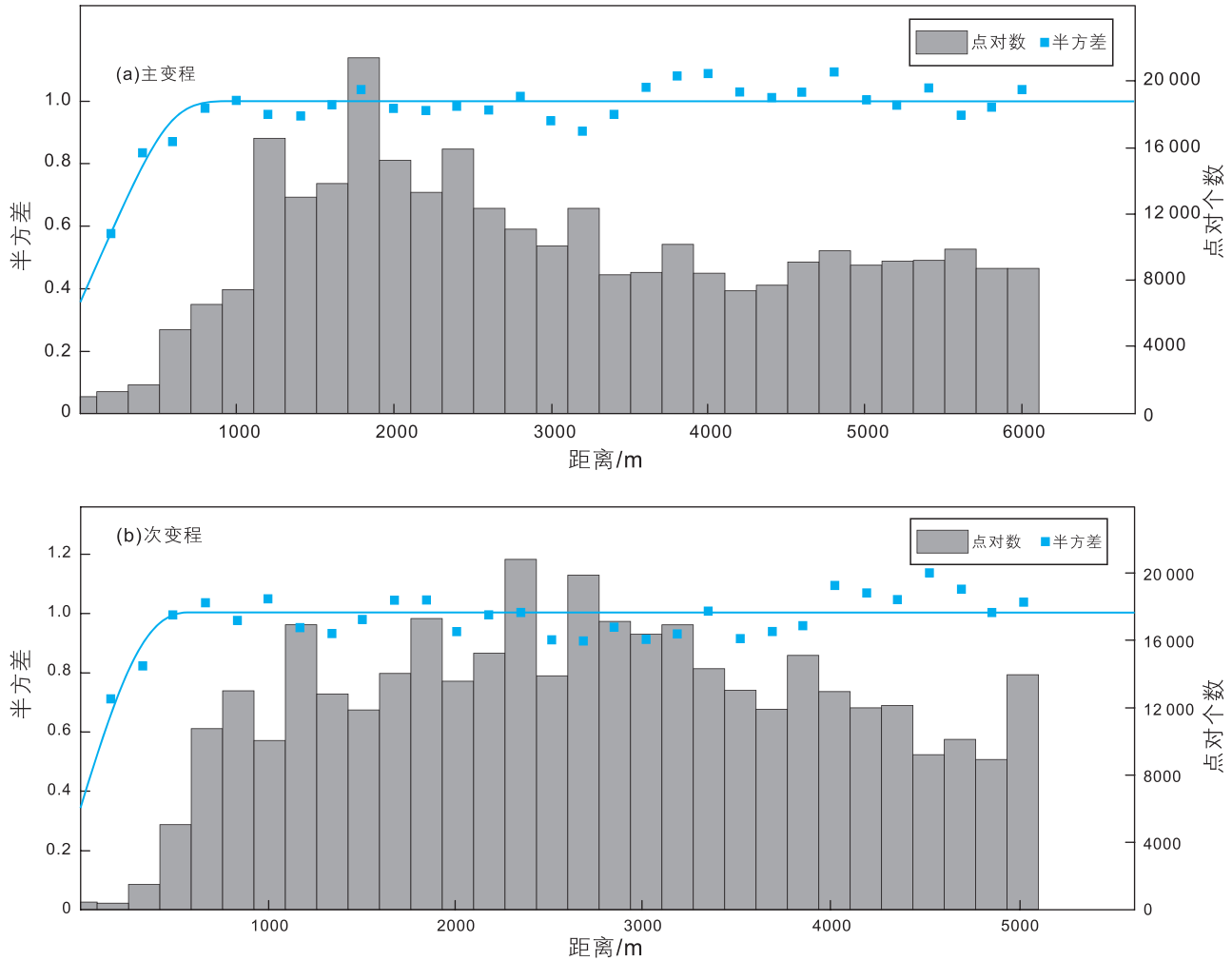
图3 水平井数据河道砂体变差函数(主变程方向 -13^\circ )
