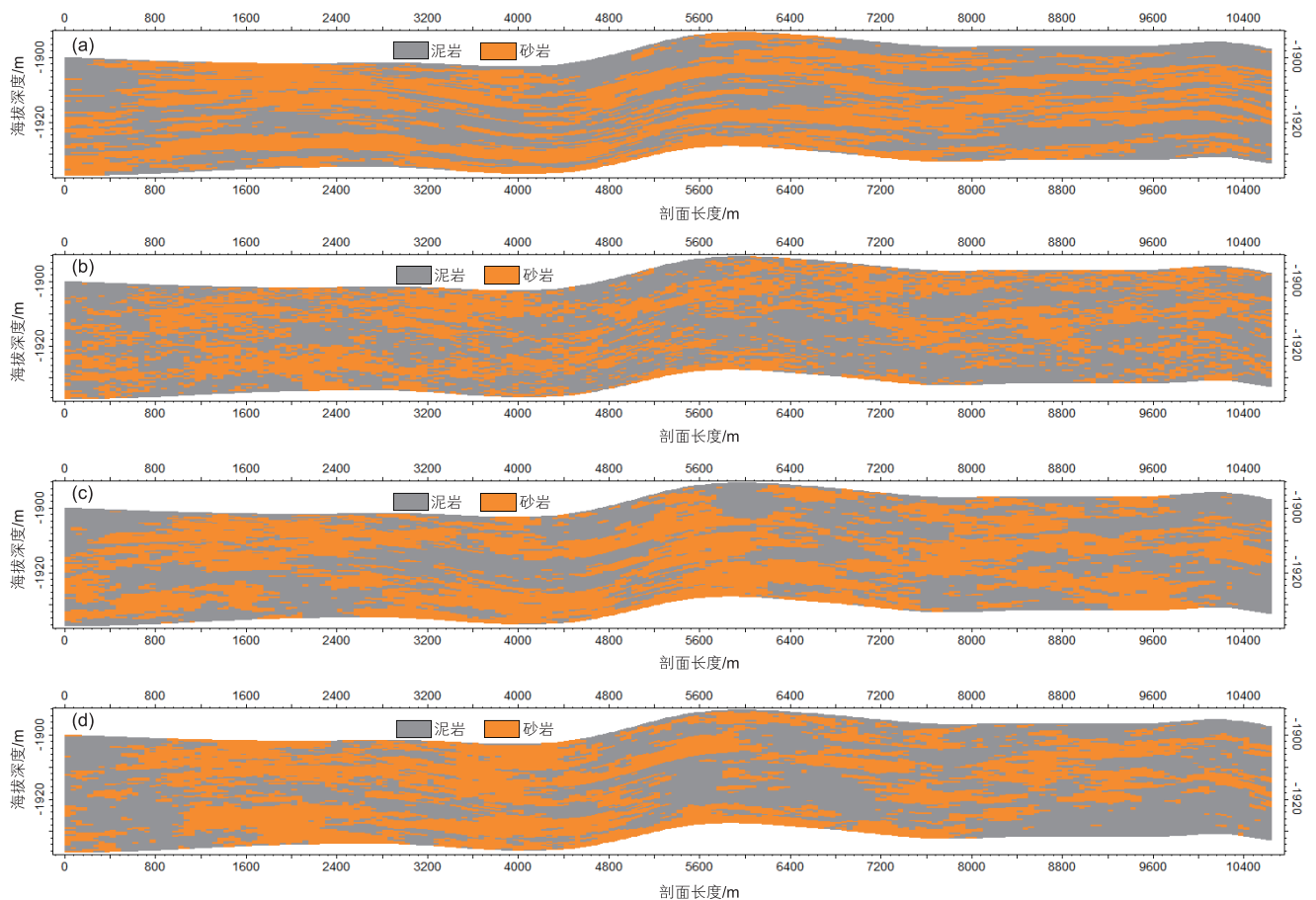
图 8 建模结果对比图 (a)直井变差函数建立的模型剖面；(b)直井加水平井变差函数建立的模型剖面；(c)变程椭圆计算法变差函数建立的模型剖面；(d)水平井段数据抽稀法变差函数建立的模型剖面
