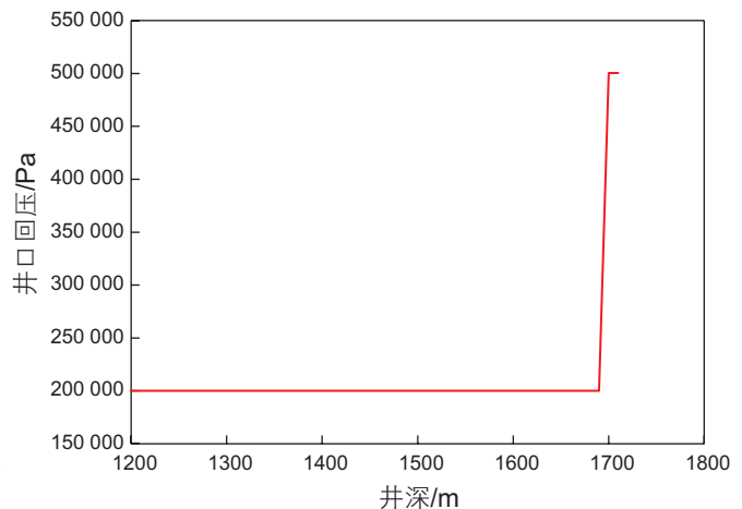
(b) 最大钻进深度为 1710 m 时对应的最优井口回压
