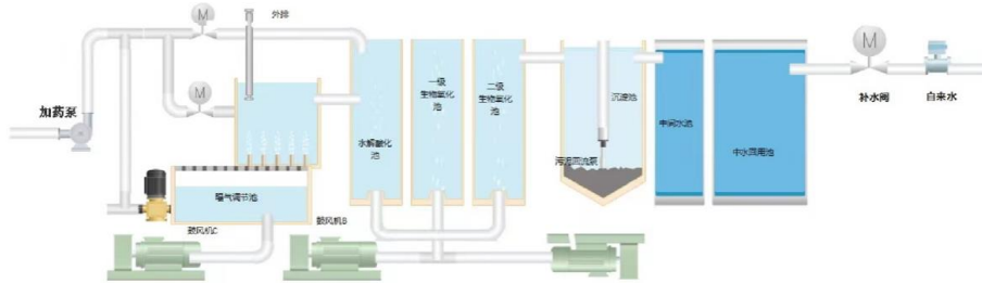
图 1 污水处理工艺流程图
