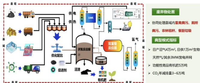
图 1 沼气工程流程示意图
